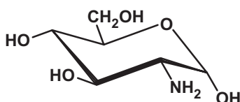
D-mannosamine
